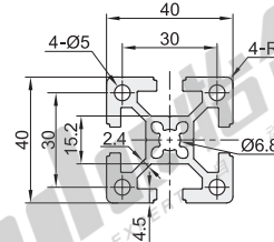
AOB05-J4040B 重量:1.42Kg/m
