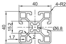
AOB05-J4040GE 重量:1.36Kg/m
