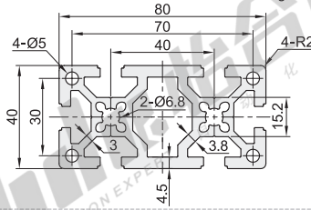
AOB05-J8840R 重量:3.23Kg/m
