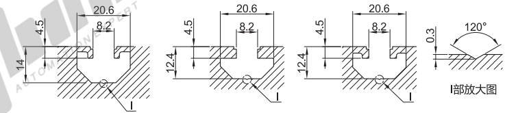
AOB05-J4040CE 重量:1.33Kg/m
