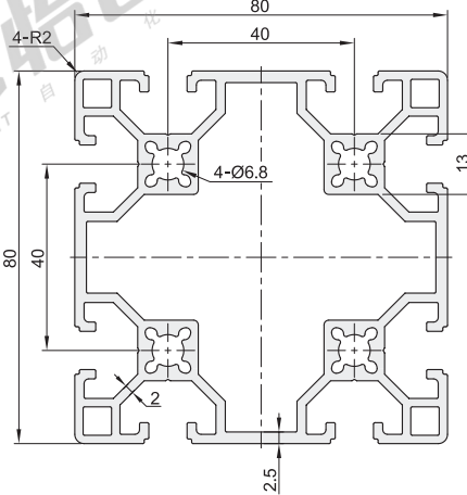
AOB05-J8080J 重量:5.53Kg/m
