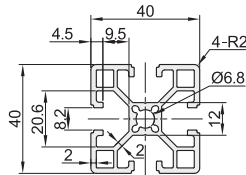
AOB05-J4040CE 重量:1.33Kg/m
