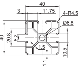
AOB05-J4040T 重量:1.42Kg/m
