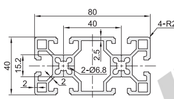
AOB05-J4080E 重量:2.7Kg/m
