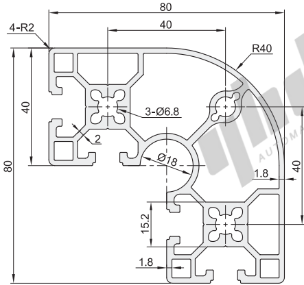
AOB05-J8840RA 重量:3.22Kg/m
