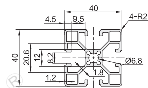
AOB05-J4040C 重量:1.18Kg/m
