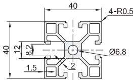
AOB05-J4040GA 重量:0.92Kg/m
