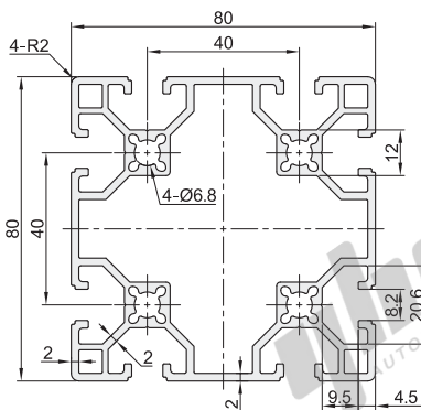
AOB05-J8080CE 重量:3.48Kg/m
