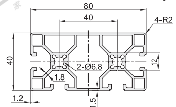
AOB05-J8840R 重量:3.23Kg/m
