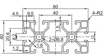
AOB05-J4080C 重量:2.04Kg/m
