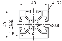
AOB05-J4040GB 重量:0.94Kg/m
