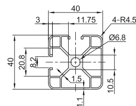
AOB05-J4040R 重量:1.25Kg/m
