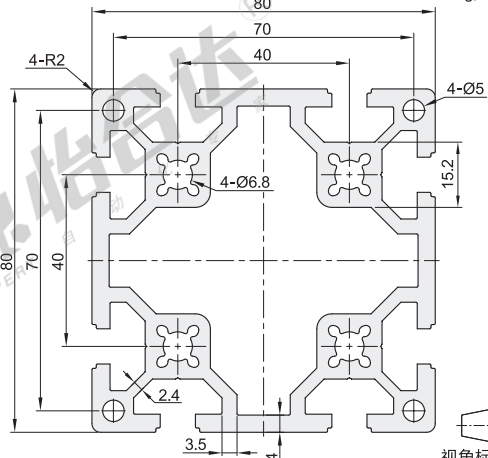
AOB05-J8080J 重量:5.53Kg/m
