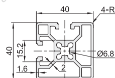
AOB05-J4040B 重量:1.42Kg/m
