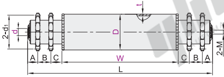
平端面型 QCH26/27
