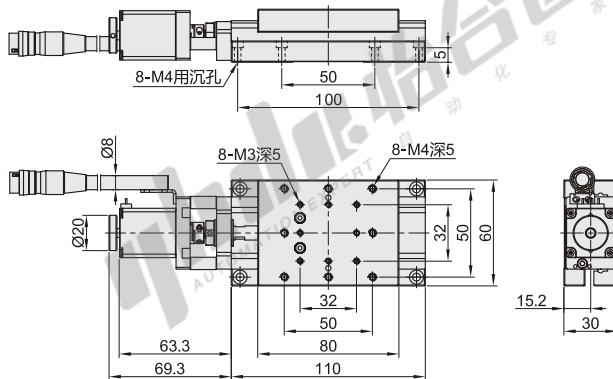
电机：MZ2C(鸣志闭环步进电机)
