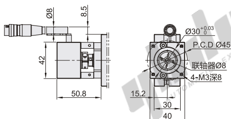
电机：U45(PCD45伺服电机座)
