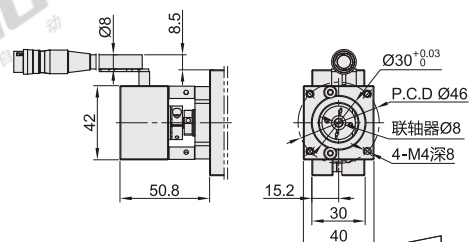
电机：U46(PCD46伺服电机座)
