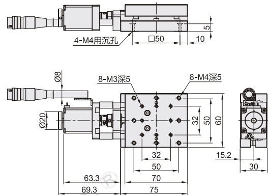
规格：6030
