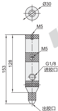
装配示意图
