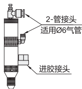
装配示意图
