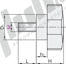
外螺纹型 HAT01
