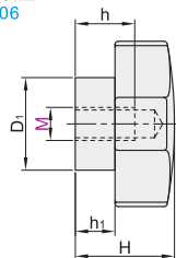
内螺纹型 HAT06
