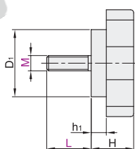
外螺纹型 HAT11
