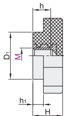
内螺纹型 HAT16
