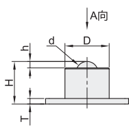
QDA20(S45C)
