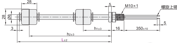
双点液位 ZJL72
