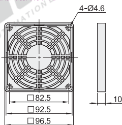
适用风扇外形尺寸: 92
