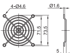
适用风扇外形尺寸: 80
