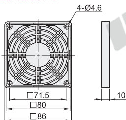
适用风扇外形尺寸: 80
