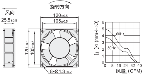
外形尺寸: 12025B
