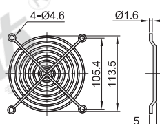
适用风扇外形尺寸: 120
