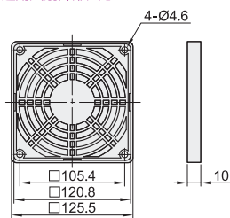
适用风扇外形尺寸: 120
