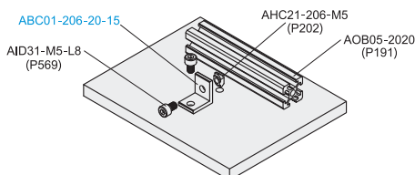
分解图
