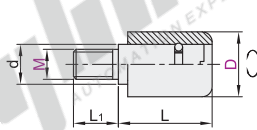
外螺纹型 HAB26
