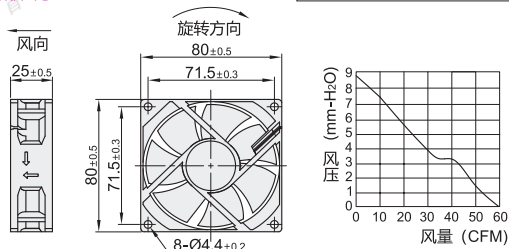
外形尺寸: 8025
