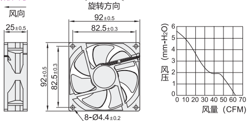
外形尺寸: 9225
