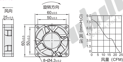
外形尺寸: 6025
