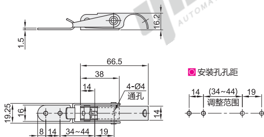
螺纹调节型 HFQ83
