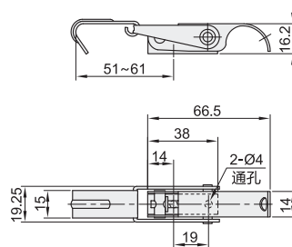
弹簧压缩型 HFQ84
