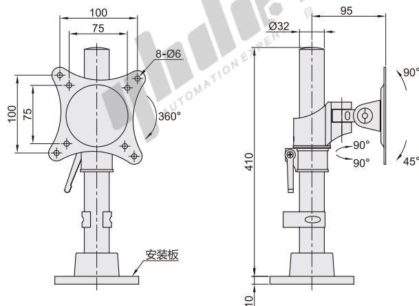
锁孔安装 NHD15
