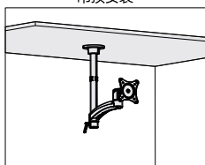
吊顶安装
