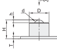
方法兰式 QDA20
