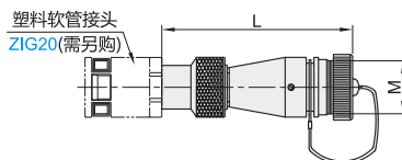
ZN(直式对接塑料软管插座)
