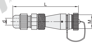
ZU(直式对接夹爪锁紧电缆插座)
