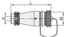
ZE(直式对接夹爪紧固插座)
