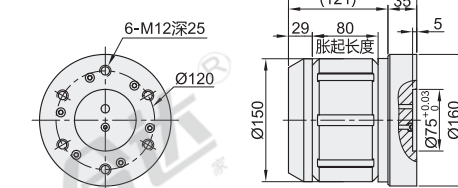
鼓皮式:双气孔
