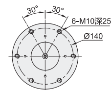
鼓皮式:普通型
