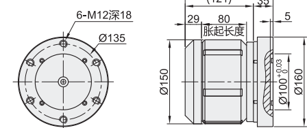
鼓皮式:气缸斜推
