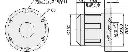
鼓皮式:双气孔
