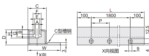
纵向型 VSW36/37
