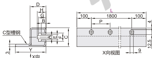
横向型 VSW31/32
