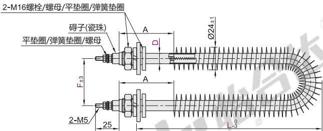
M16螺栓
