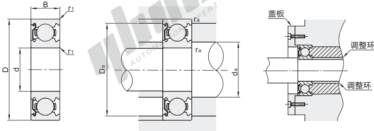
安装图
