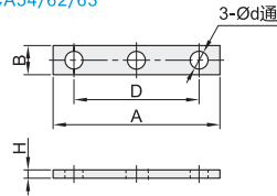
扁平式护套用 VCA54/62/63
