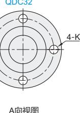
圆法兰式 QDC32
