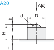
方法兰式 QDA20
