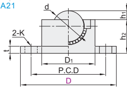
圆法兰式 QDA21
