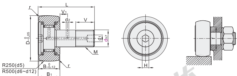
球面型 BPP05
