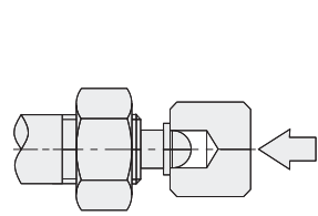
油嘴安装方法
