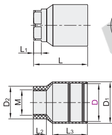
立柱管接头 ZCD23
