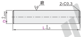
标准型·直杆型 Y-GAF02
