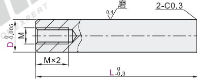
标准型·一端内螺纹型 Y-GAF12
