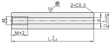
管型·一端内螺纹型 Y-GAJ12
