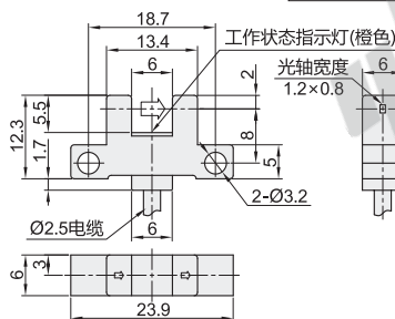
ZJF49-F25-N/P
