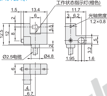
ZJF49-F25-N/P
