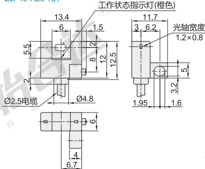
ZJF49-R25-N/P
