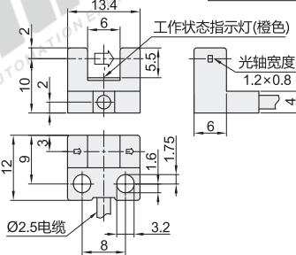
ZJF49-R25-N/P
