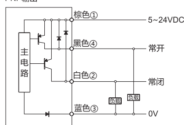
PNP输出
