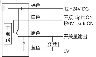
PNP输出
