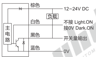
NPN输出
