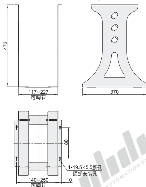
吊顶安装 ZCA41
