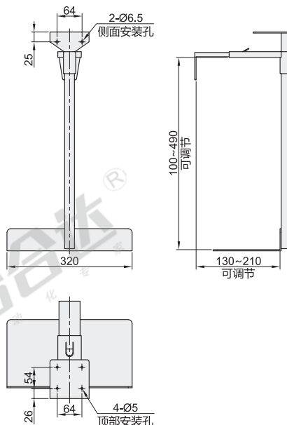
吊顶安装/壁挂式安装 ZCA42
