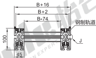
A-A放大图
