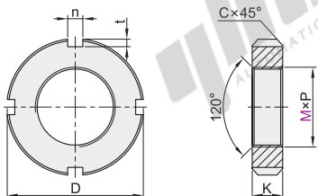
小圆螺母 TBK71
