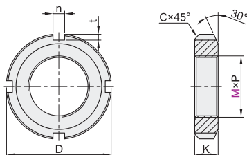
圆螺母 TBK74 TBK75
