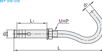
有缝小头膨胀钩 TBF58/59
