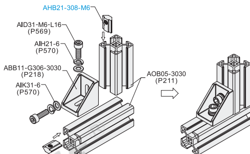
分解图
