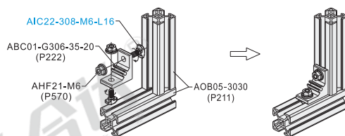
分解图
