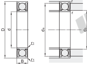
安装图
