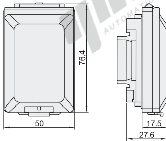
外形尺寸
