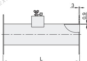
法兰型 BMG51
