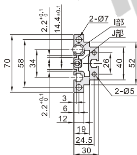
型材截面放大图 传送侧面
