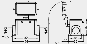
结构2: M/PG=M20/PG16使用结构2
