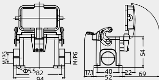
结构2：M/PG=M20/PG16使用结构2
