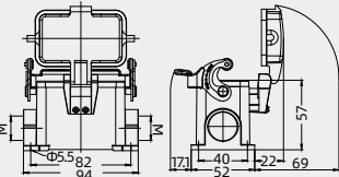
1)：结构1（M=M25使用结构1）
