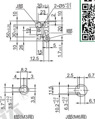
型材截面放大图
