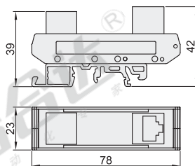
规格：TH(卧式转端子)
