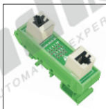
规格：H(一对一卧式)
