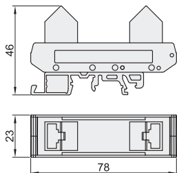
规格：TV(立式转端子)
