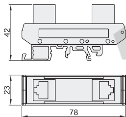
规格：A(一对一斜插)
