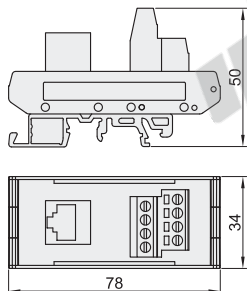
规格：TV(立式转端子)
