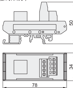
规格：TH(卧式转端子)
