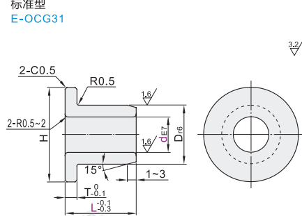
标准型 E-OCG31
