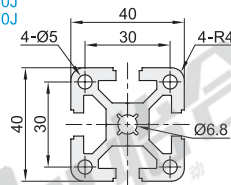
AOB05-4040A
