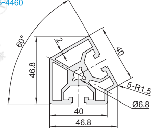
AOB05-4460
