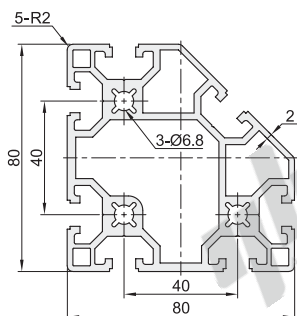
AOB05-8080XE
