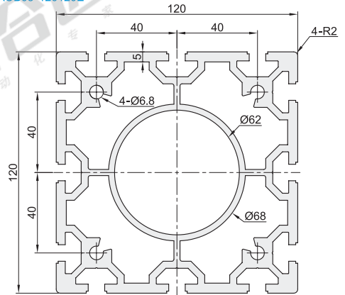
AOB05-120120E
