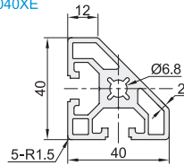
AOB05-4040XE
