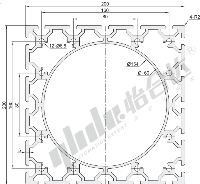
AOB05-200200E
