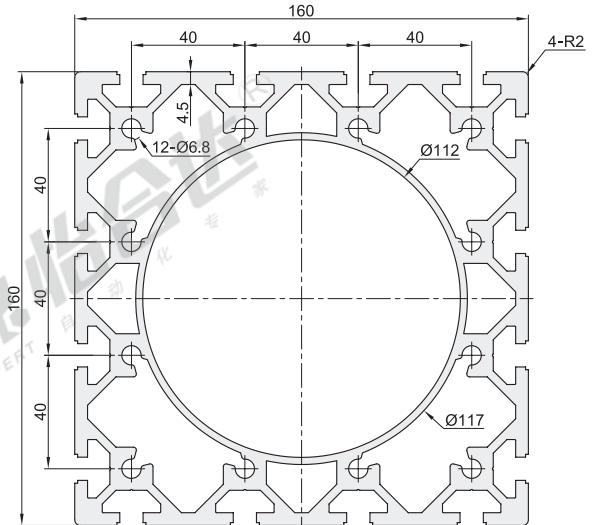
AOB05-160160E
