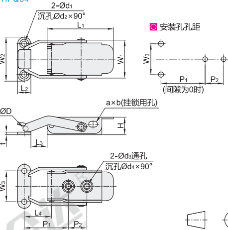
普通型 HFQ54
