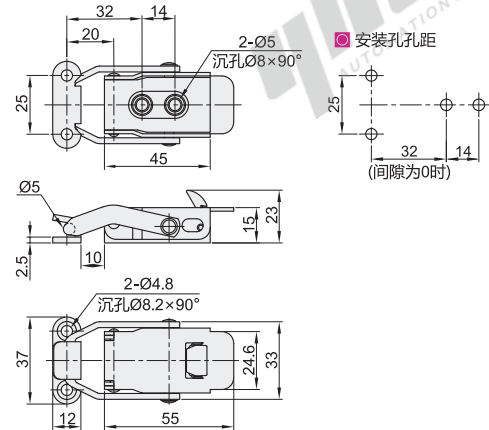
自锁型 HFQ55
