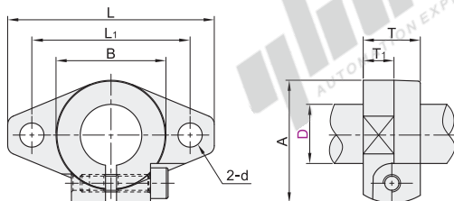
法兰型 GFC01
