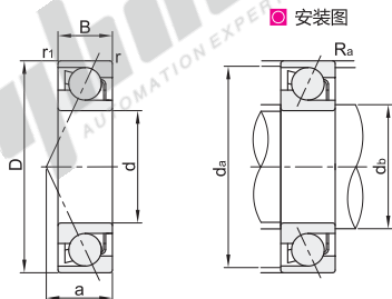
安装图
