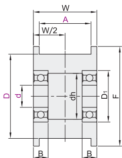
带法兰型
