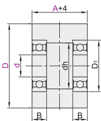
无法兰型
