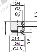
盘径 \varnothing 4
