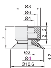
盘径 \varnothing 10
