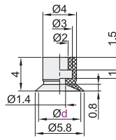
盘径 \varnothing 5
