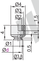
盘径 \varnothing 3.5
