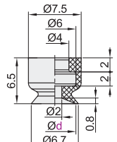
盘径 \varnothing 6
