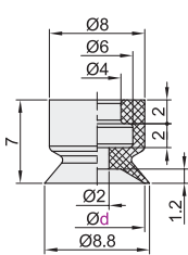
盘径 \varnothing 8
