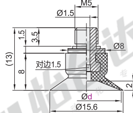
盘径 \varnothing 15
