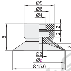
盘径 \varnothing 15
