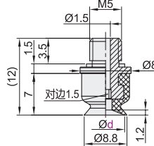
盘径 \varnothing 8
