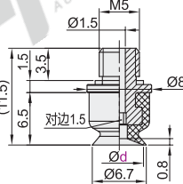
盘径 \varnothing 15
