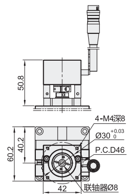
电机：U46(PCD46伺服电机座)
