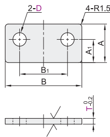
双孔型 BLC83/84
