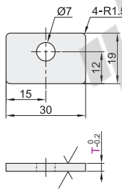
单孔型 BLC81/82
