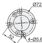
K向视图
