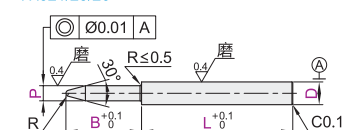
L尺寸指定型·锥头R型 YHJ21/25/26
