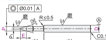
L尺寸指定型·锥角型 YHJ31/35/36
