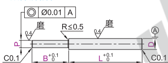
L尺寸指定型·平头型 YHJ01/05/06
