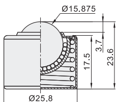
标准型 QDB01-15
