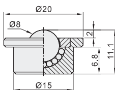
重型 QDB06-8
