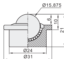
重型 QDB06-15
