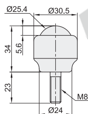
螺栓型 QDA13
